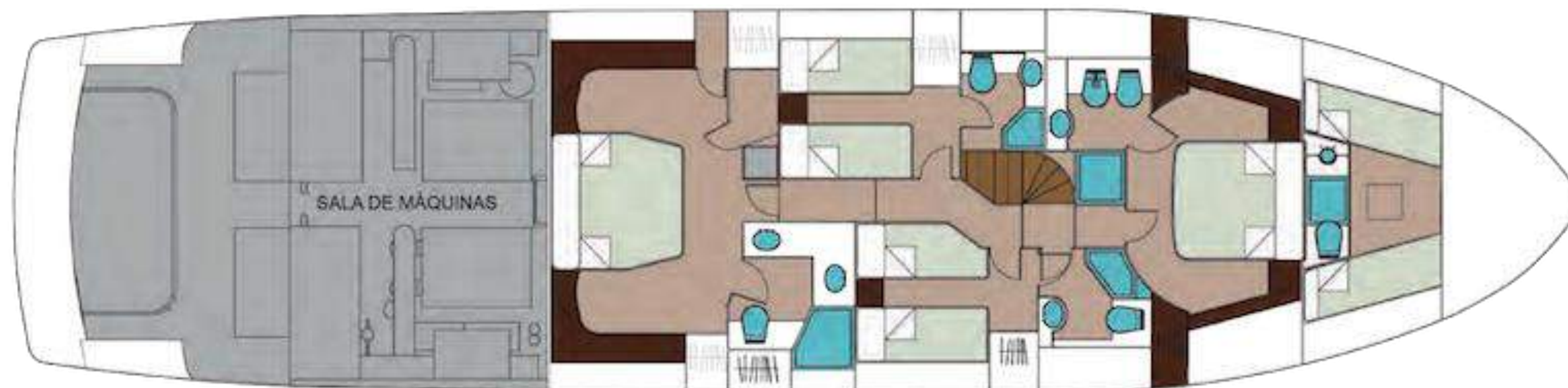
CUBIERTA INFERIOR
